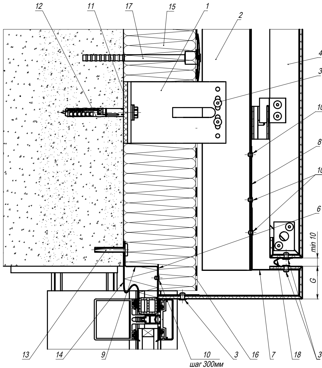
Схема расположения компонентов противопожарной отсечки
